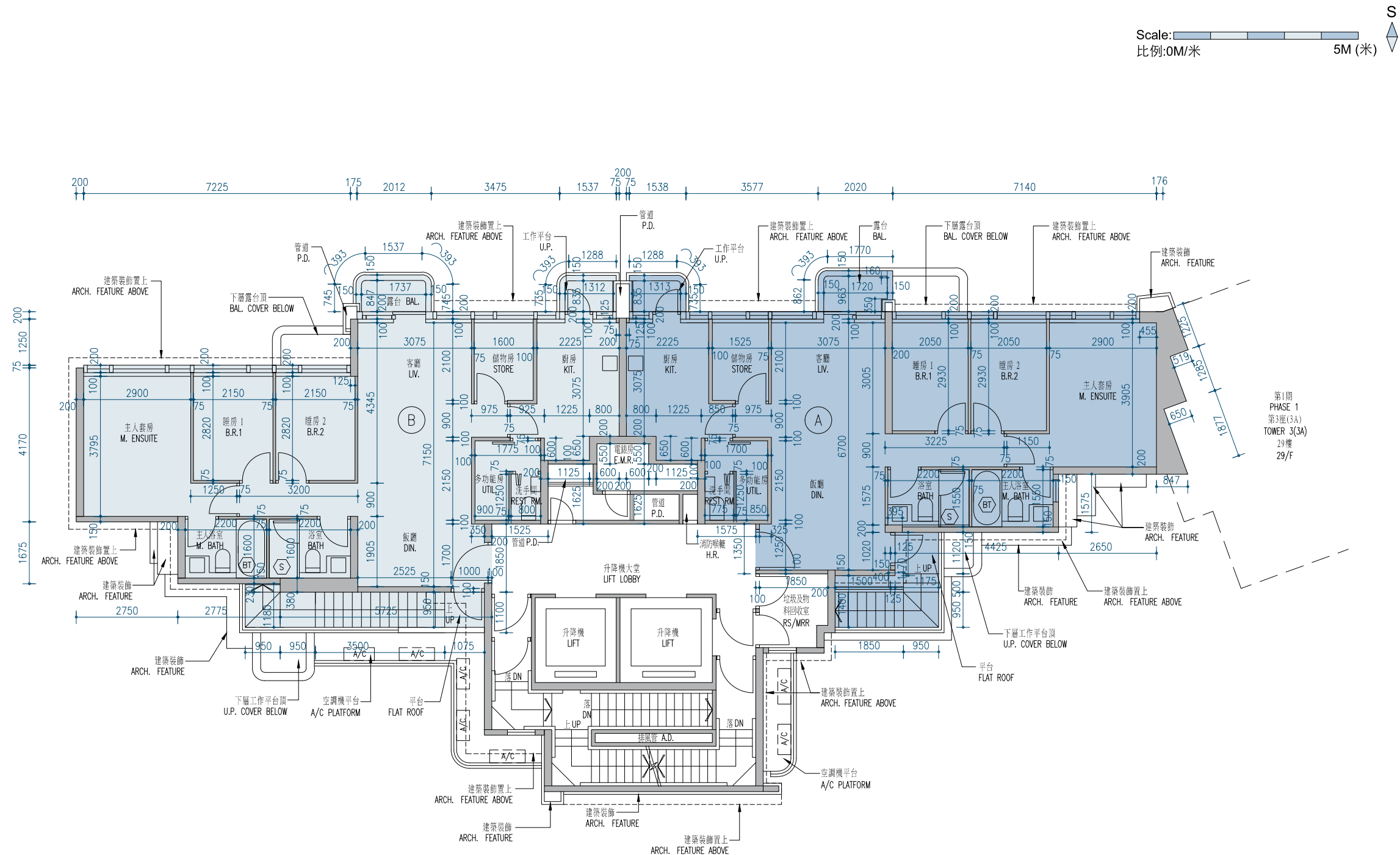
Phase 1 Tower 5 29/F Floor Plan 第1期 第5座29樓樓面平面圖
