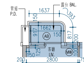
7/F-12/F, 15/F-20/F Unit A Part Plan 7樓至12樓、15樓至20樓 A單位之部分平面圖
