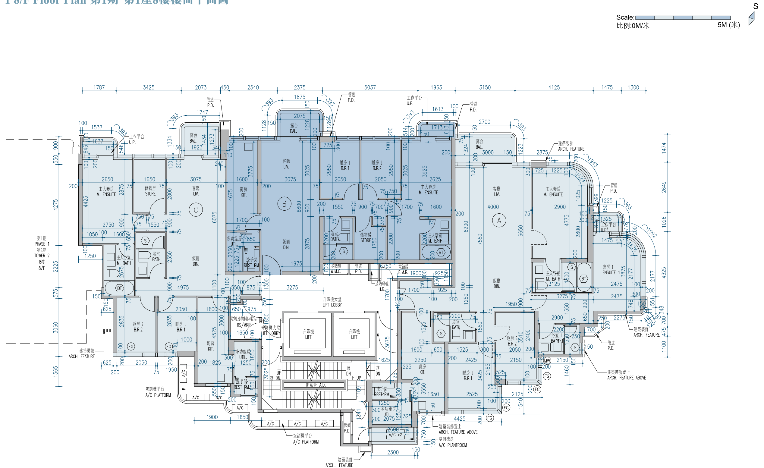
Phase 1 Tower 1 8/F Floor Plan 第1期 第1座8樓樓面平面圖
