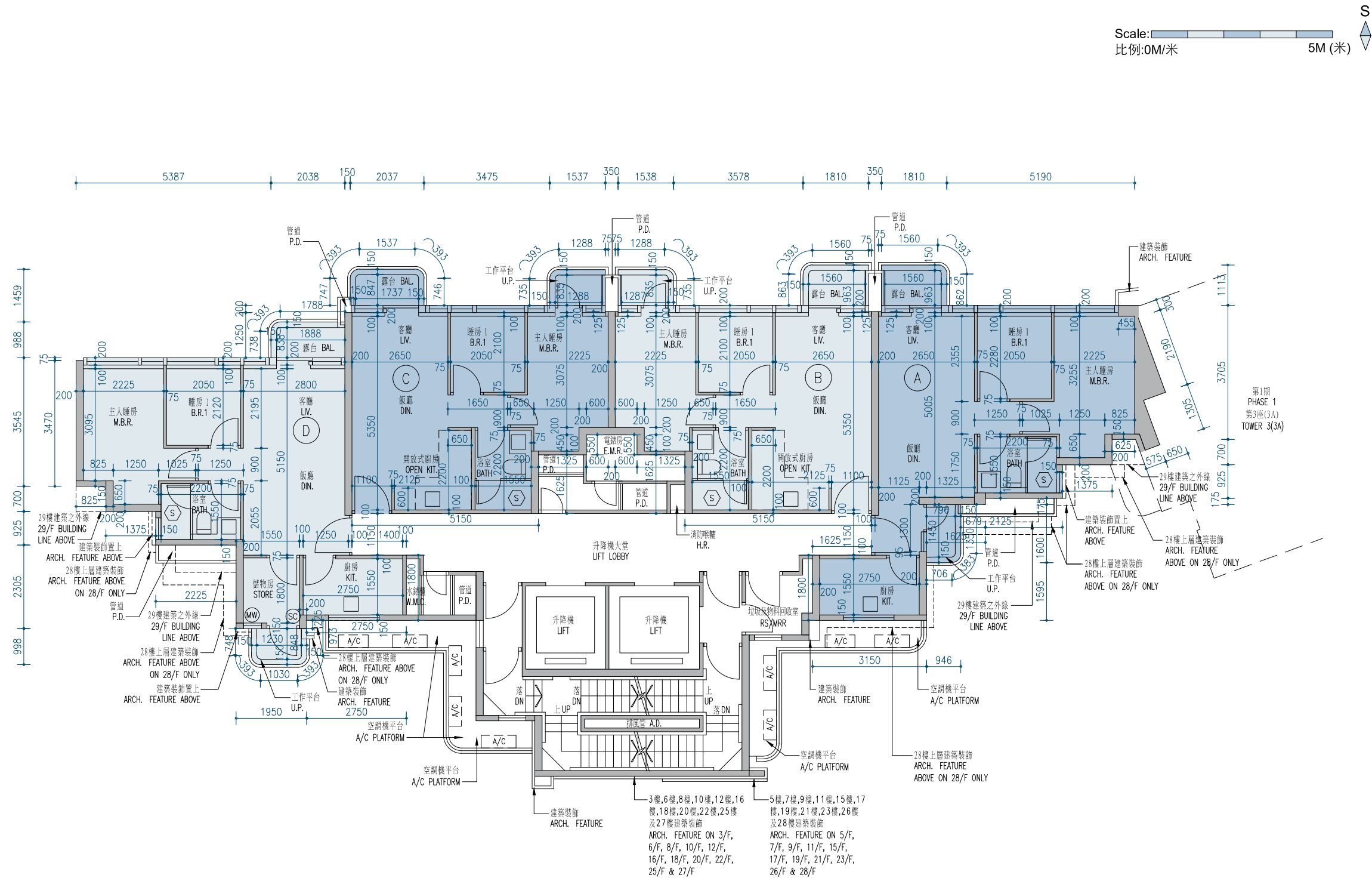
Phase 1 Tower 5 3/F, 5/F-12/F, 15/F-23/F, 25/F-28/F Floor Plan 第1期 第5座3樓、5樓至12樓、15樓至23樓、25樓至28樓樓面平面圖
