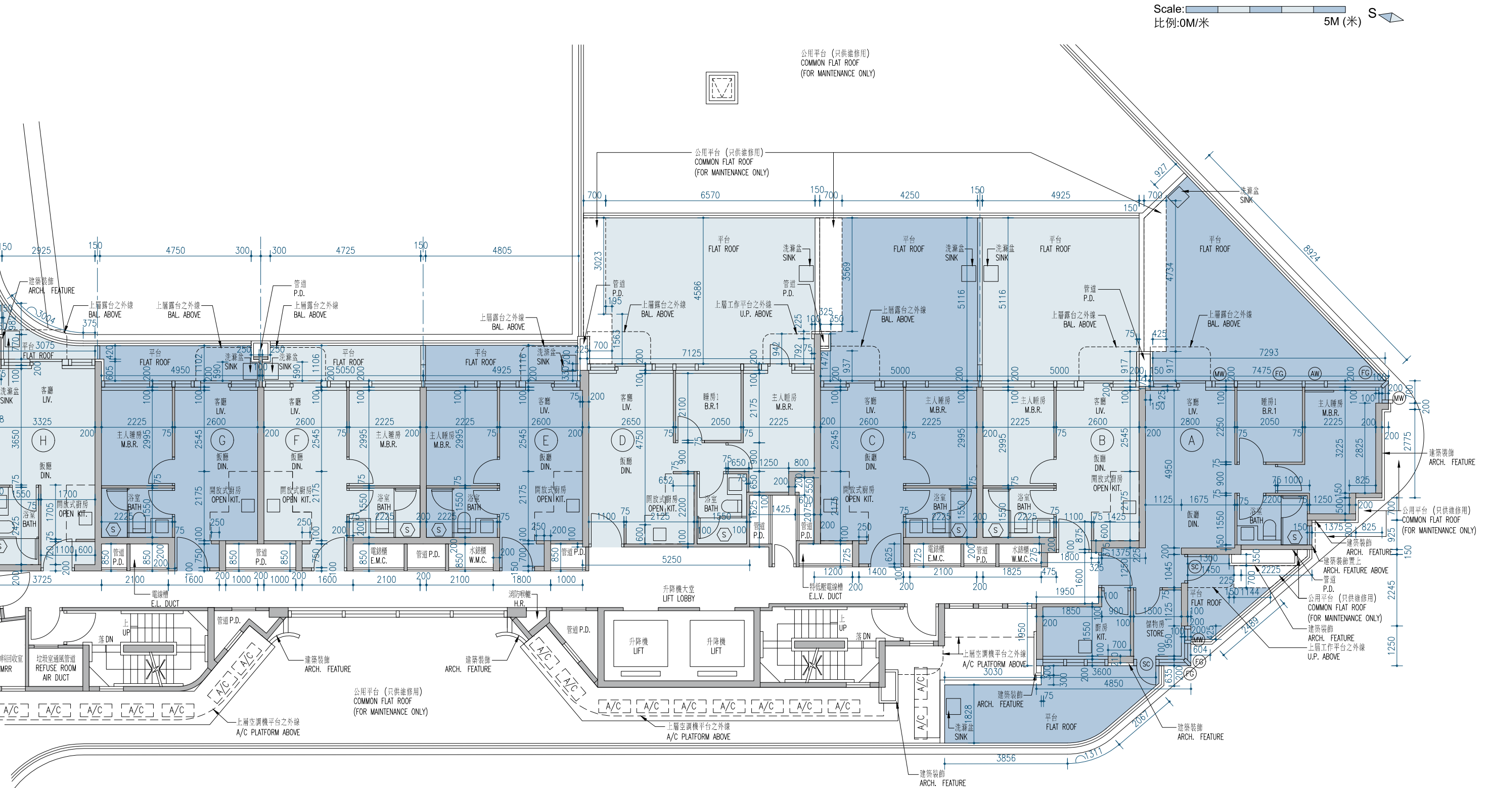
Phase 1 Tower 3(3B) 2/F Floor Plan 第1期 第3座(3B) 2樓樓面平面圖
