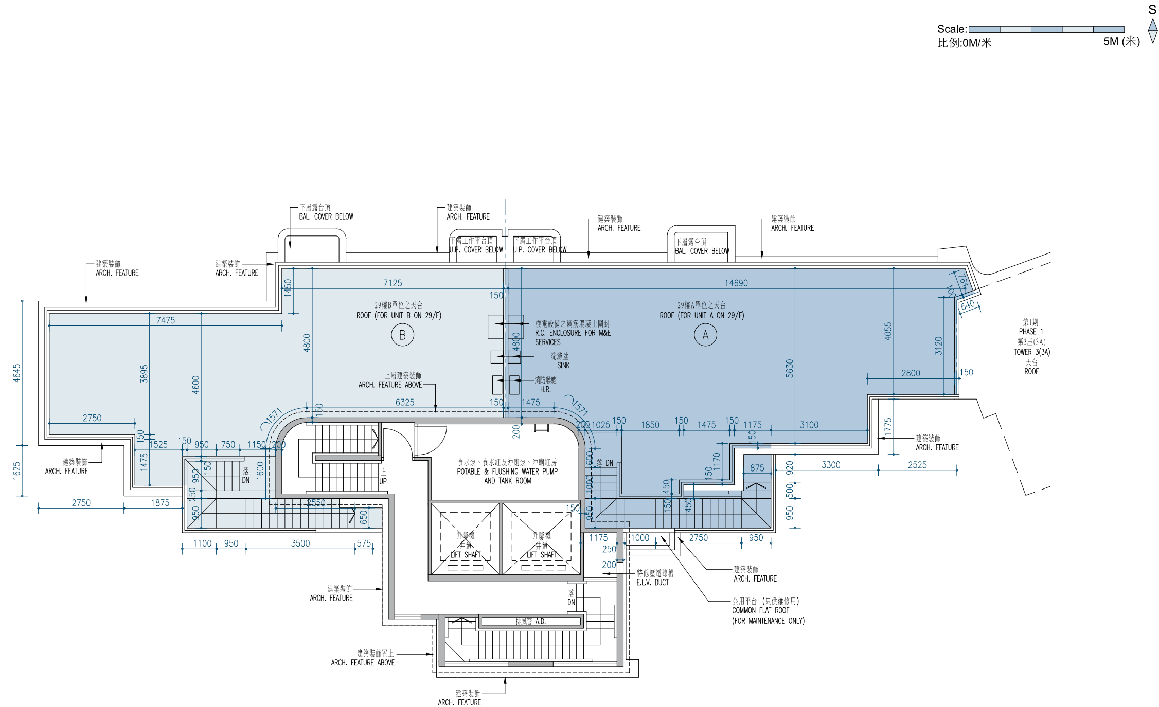
Phase 1 Tower 5 Roof Plan 第1期 第5座天台樓面平面圖
